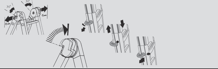
Apertura scala | Ladder opening | Ouverture de l'échelle | Posicionamiento de la escalera | Abertura da escada
